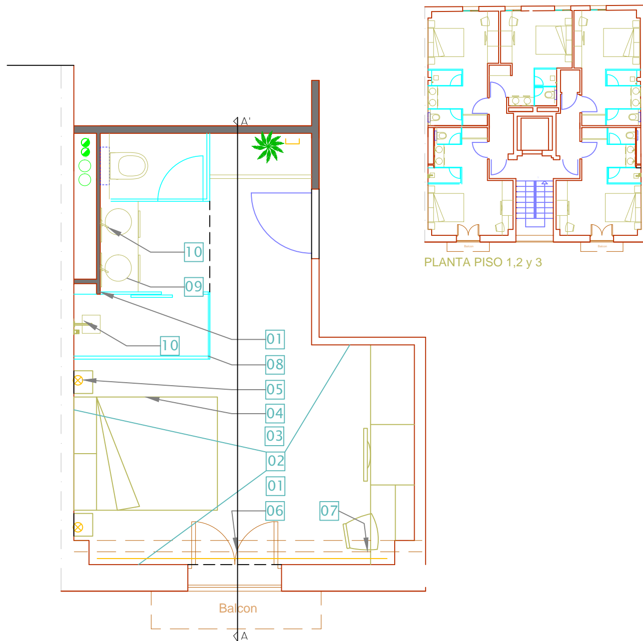
Planta Habitación Tipo
