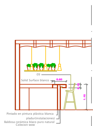
Seccion Barra bar B-B'
